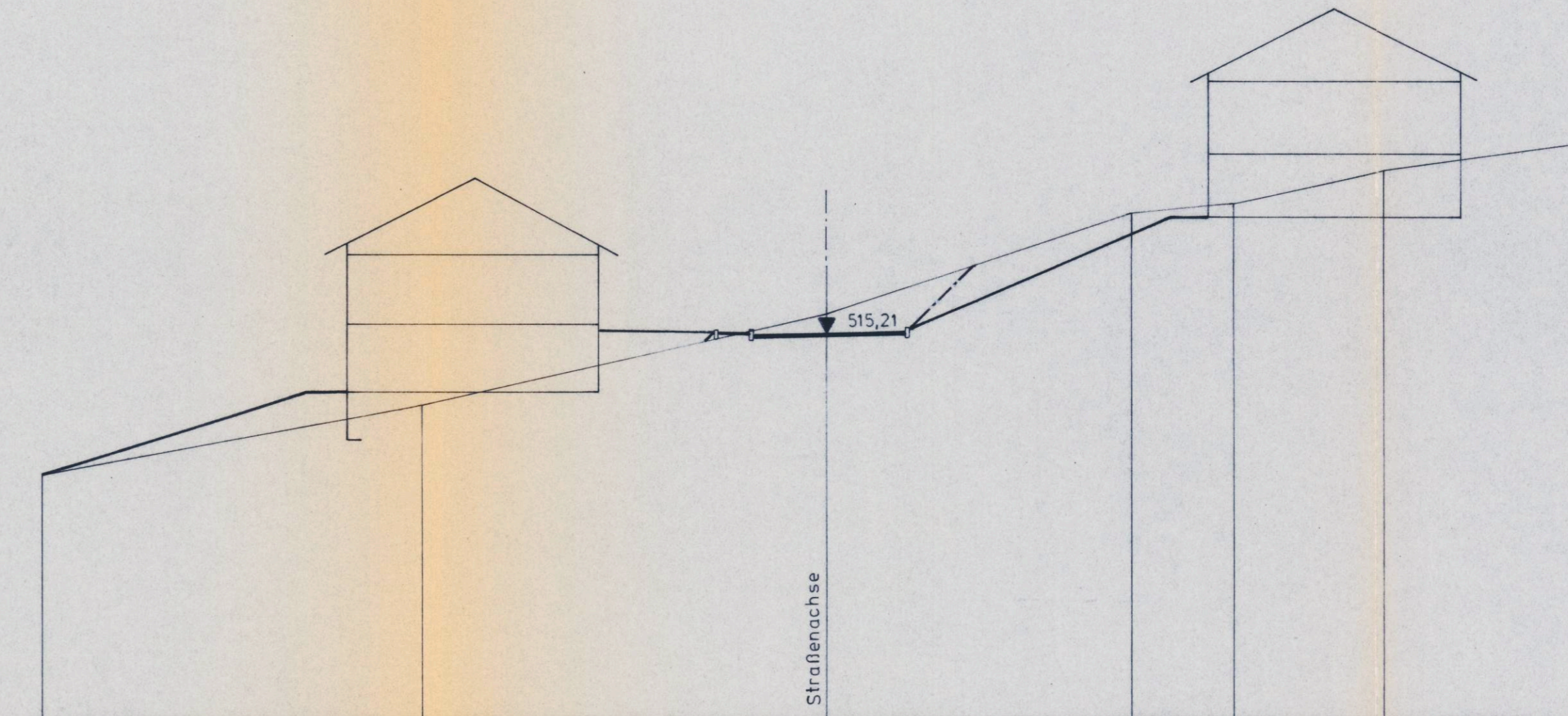
Querschnitt II-II
